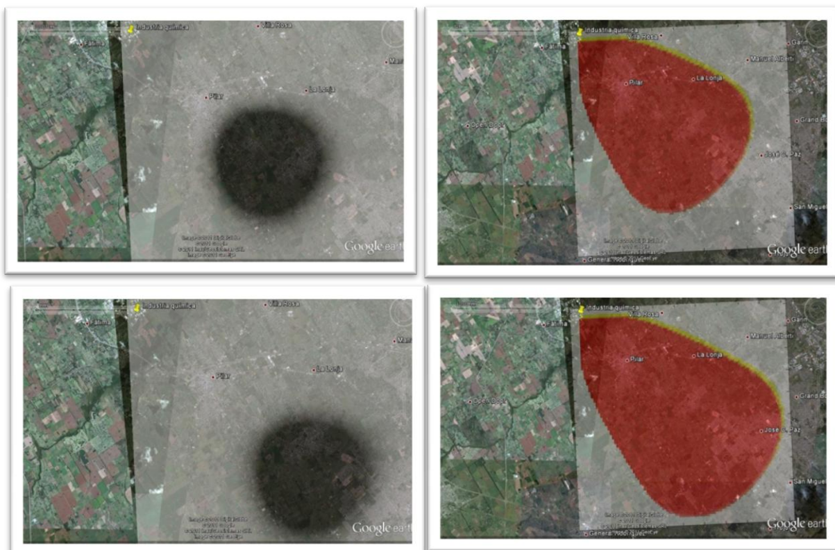
Figura 3: Representación de la evolución de la nube tóxica (PRIMERA COLUMNA) y de las regiones de daño maximal (SEGUNDA COLUMNA) para el escape en el parque industrial de pilar, EN los tiempos de SIMULACIÓN DE 120 (arriba) y 180 (abajo) minutos. FUENTE: GOOGLE EARTH, 2011.
