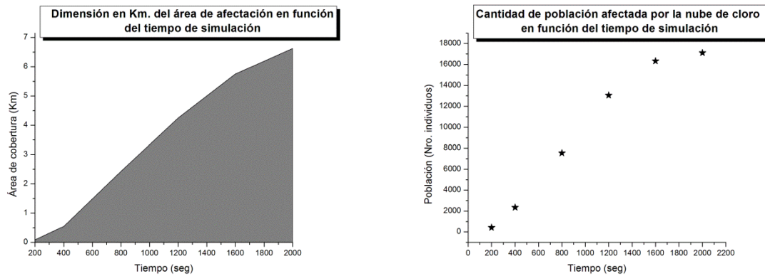
Figura 2: Análisis de la dimensión de las regiones de afectación y de la cantidad de población afectada en función del tiempo de simulación.
